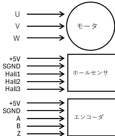
エンコーダ ハーネス 配色
